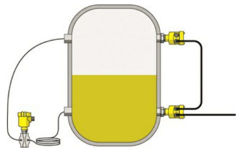
传统式(左)和电子式(右)压差测量法
