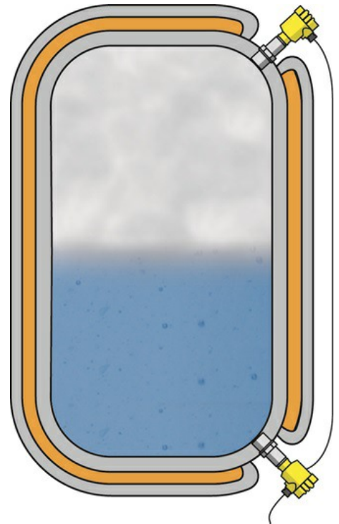
为实现远距离供热在一个补偿容器上进行电子式压差测量
